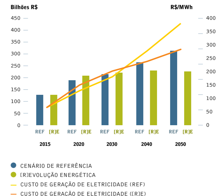
figura 6.7: evolução dos custos totais de fornecimento de eletricidade e custos de geração por MWh em ambos os cenários
